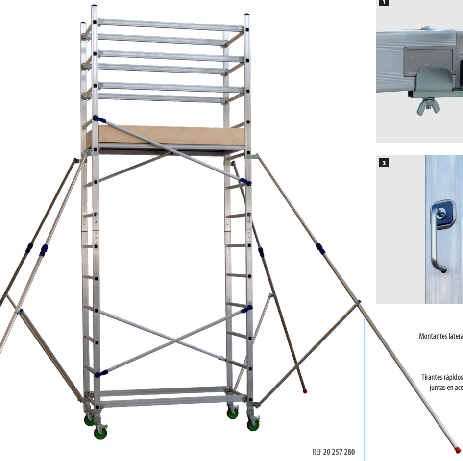
1 Enganches de seguridad en aluminio fundido.
