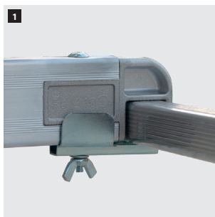
1 Enganches de seguridad en aluminio fundido.
