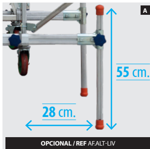
A Niveladores regulables horizontal y verticalmente.
