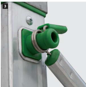
3 Bloqueo rápido de las diagonales con exclusivos muelles de acero inoxidable.
