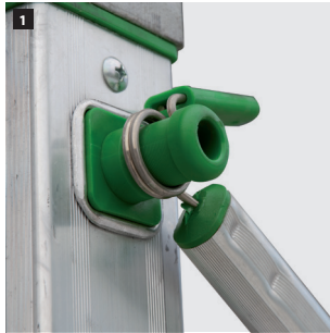
1 Bloqueo rápido de las diagonales con exclusivos muelles de acero inoxidable.
